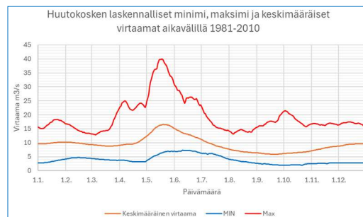
Huutokosken virtaamat 1981–2010. Kuva: P-S ELY-keskus
