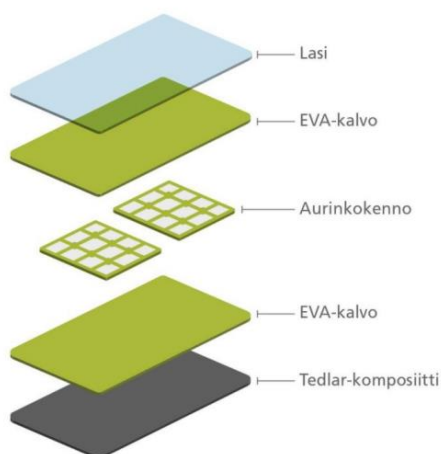
Kuva 8. Aurinkopaneelin kerrosrakenne
