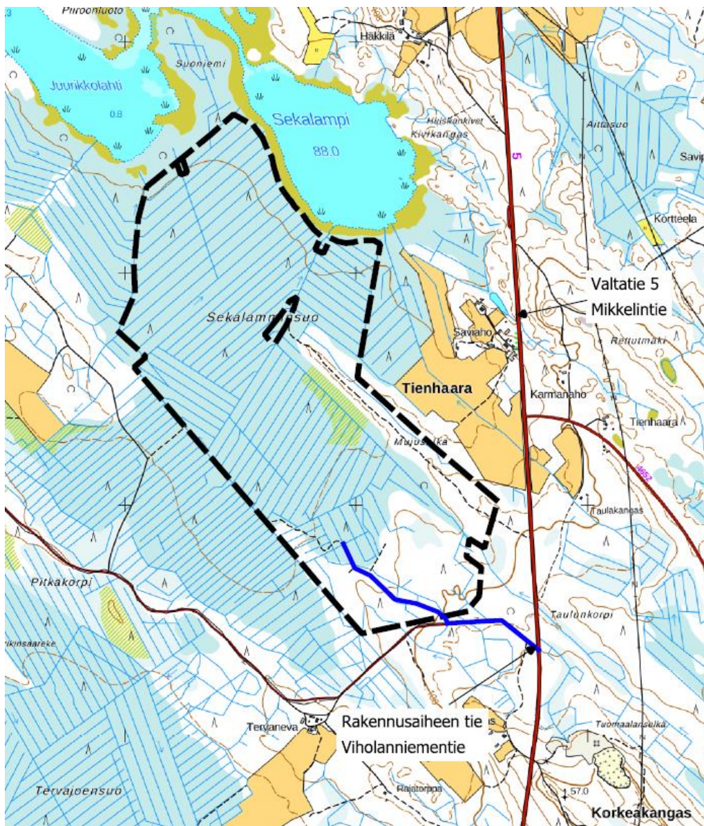
Kuva 4. Aurinkovoimalan rakennusvaiheen tiestö.
