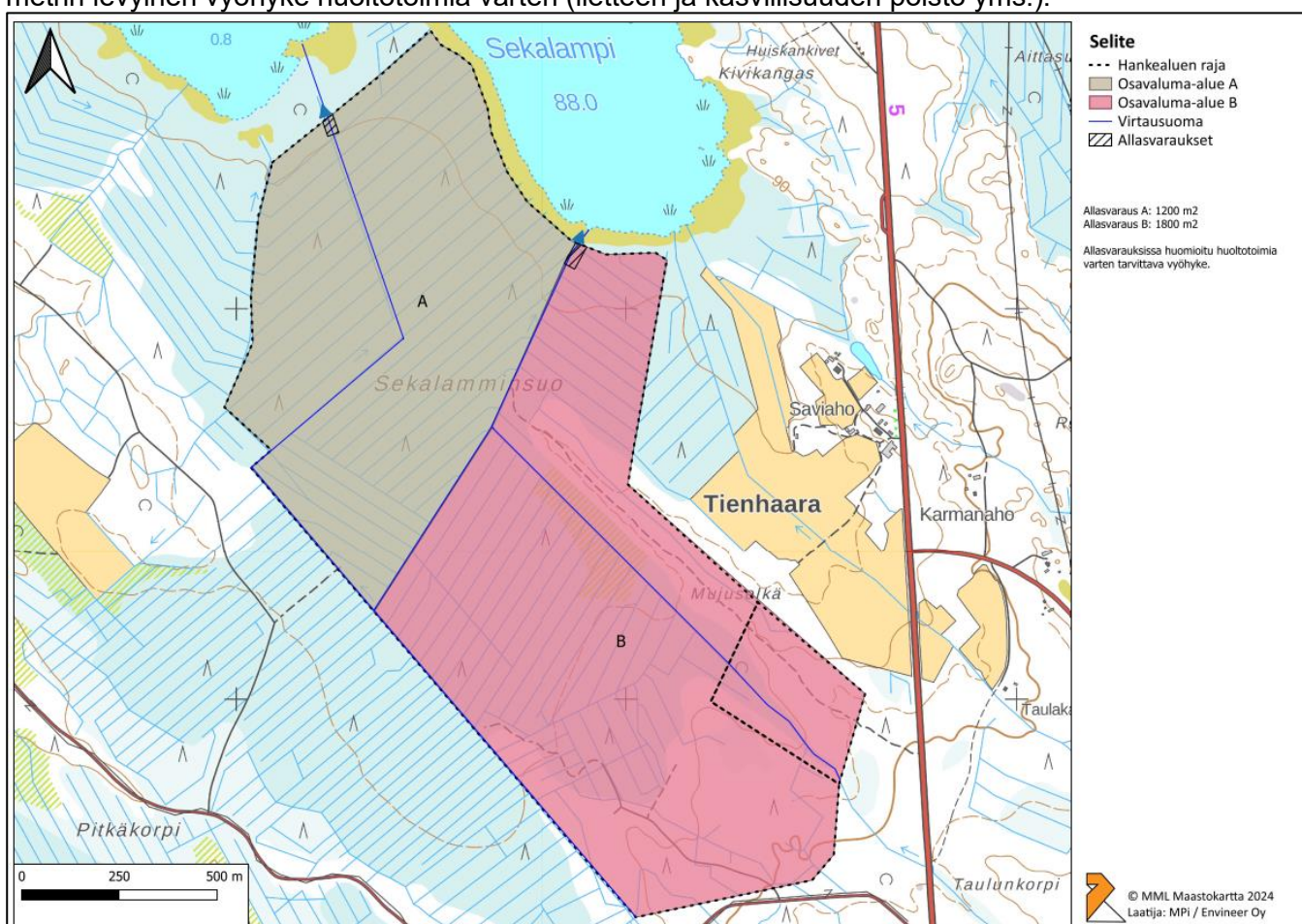
Kuva 10. Hankealueen osavaluma-alueet ja valumavesien purkupisteet ja viivästysallasvaraukset
