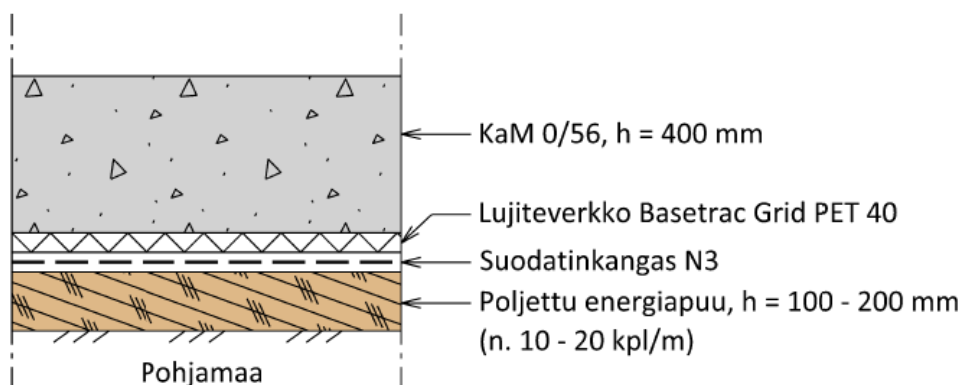
Kuva 5. Alustava poikkileikkaus suolle tehtävien teiden rakenteesta.
