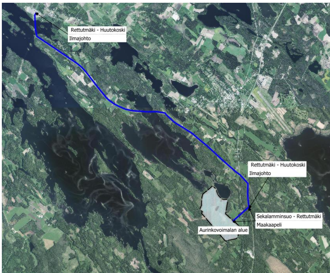
Kuva 6. Sähköliittymän alustava linjaus.
